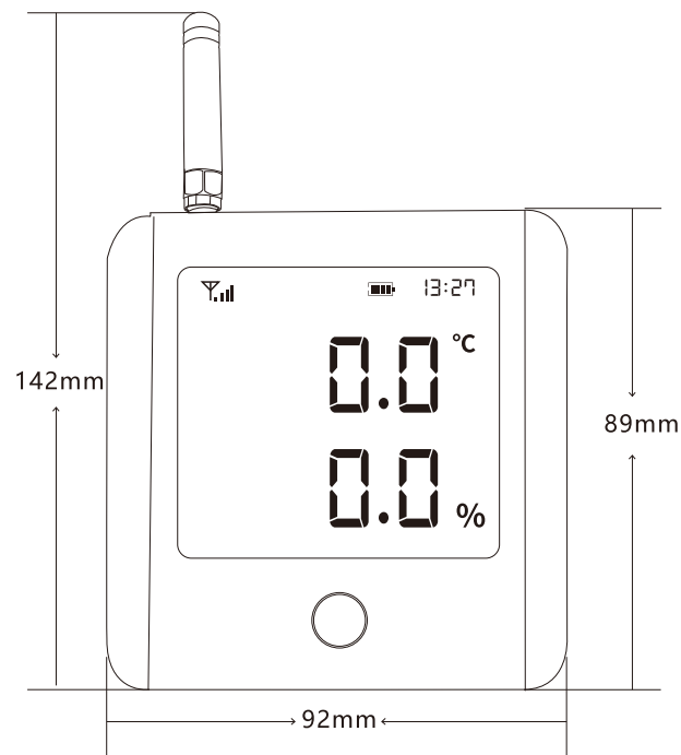
正视图
